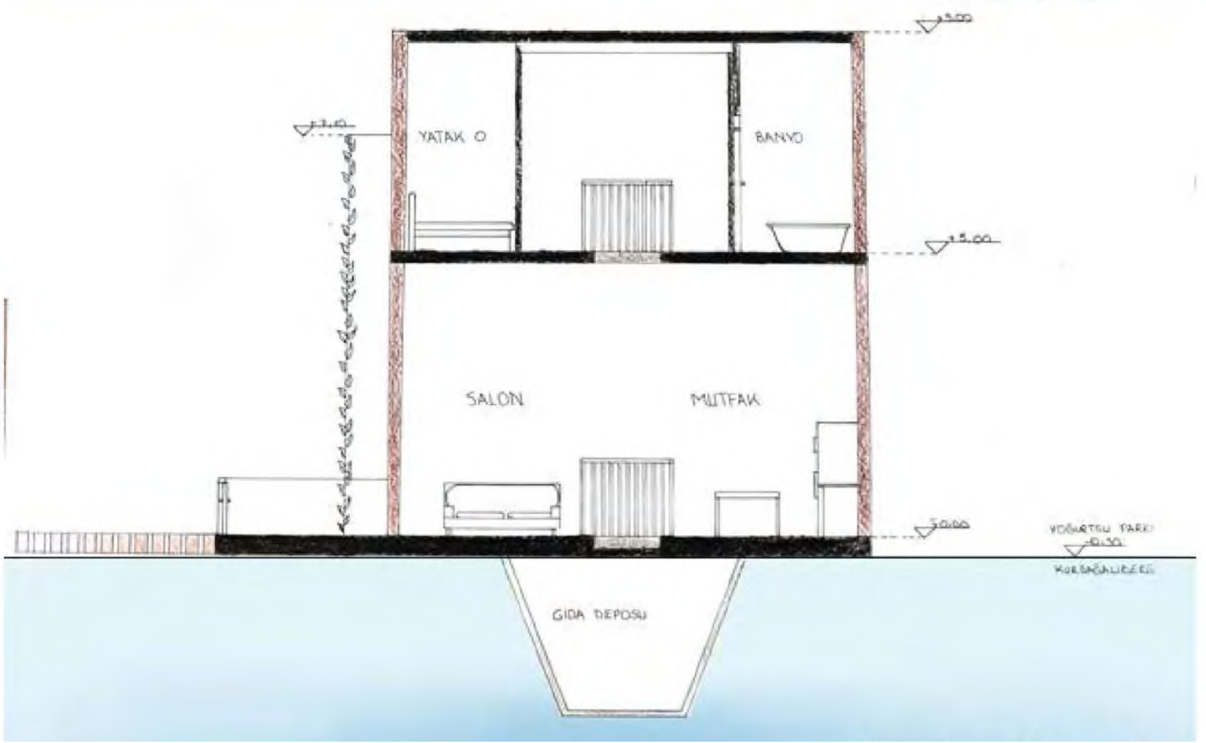
150 YAKIN A-A KESİTİ 1/50 ÖLÇÜLÜ B-B KESİTİ
